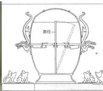
图 2-5-12 候风地动仪的构造
